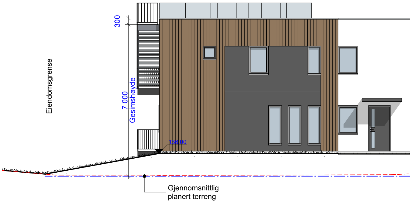
1:100 Fasade Øst
