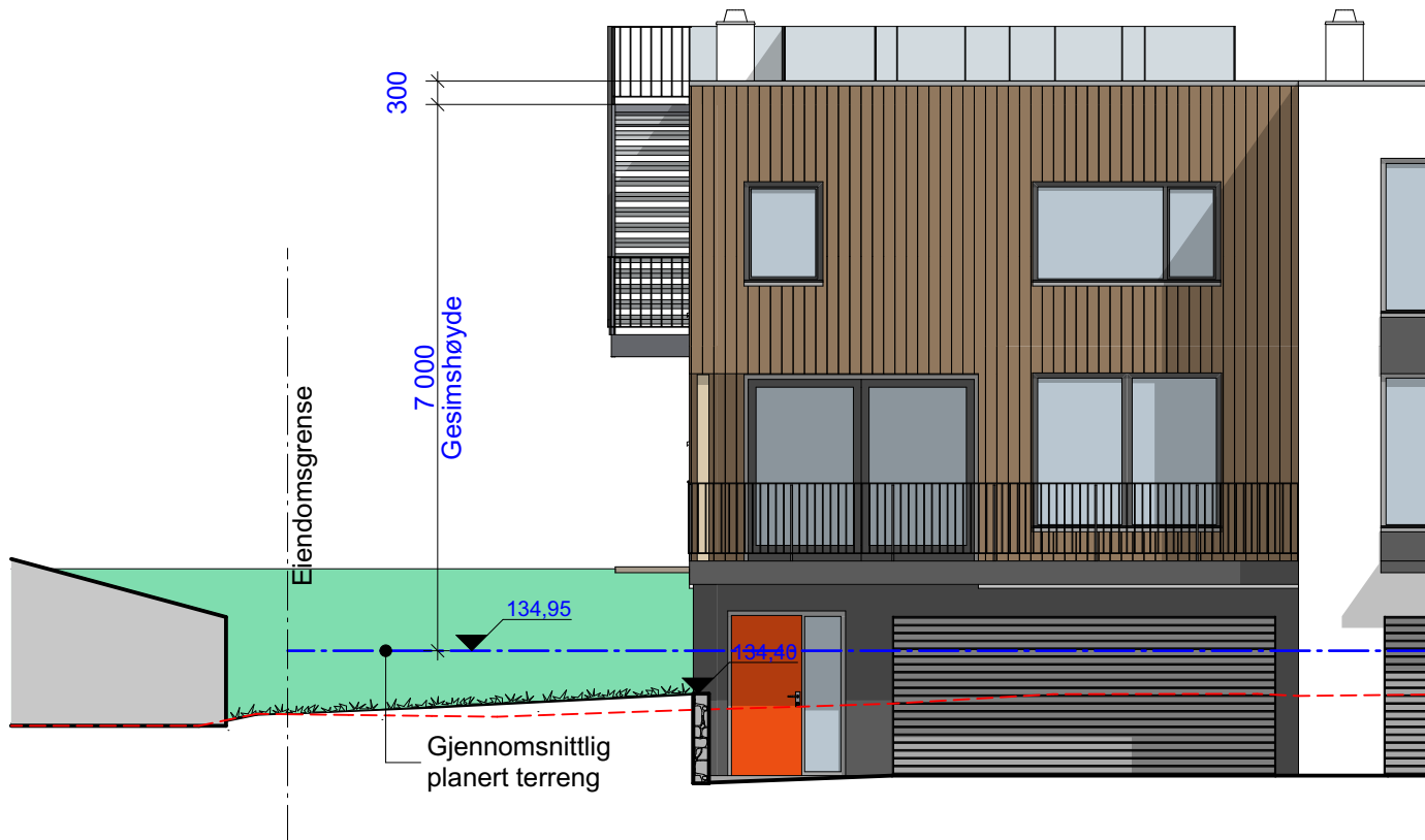
1:100 Fasade Vest
