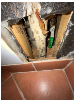
Vann- og avløpsrør. Stoppekran.
