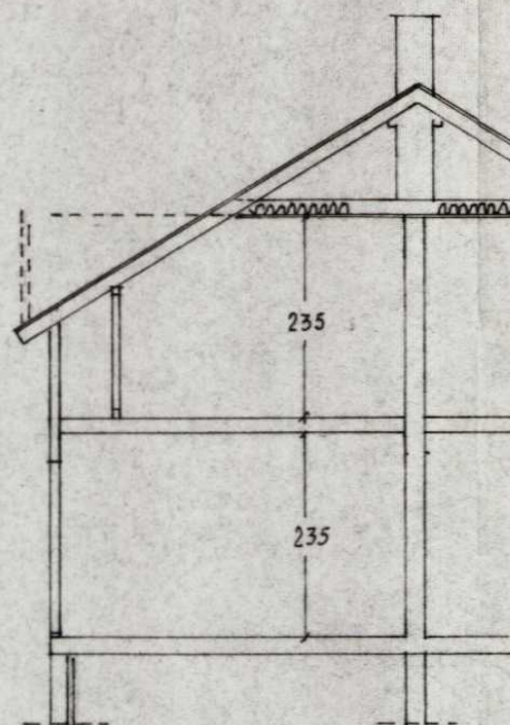
SNITT A-A
